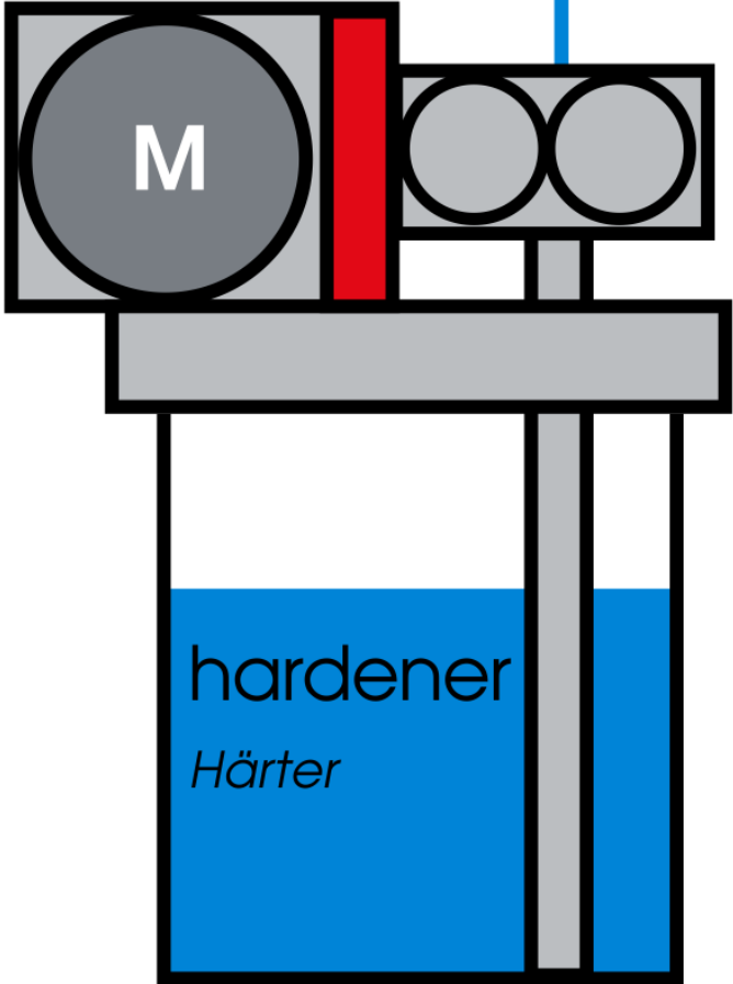
Sealless metering pump Frequenzgeregelte, leakagefreie Dosierpumpe
